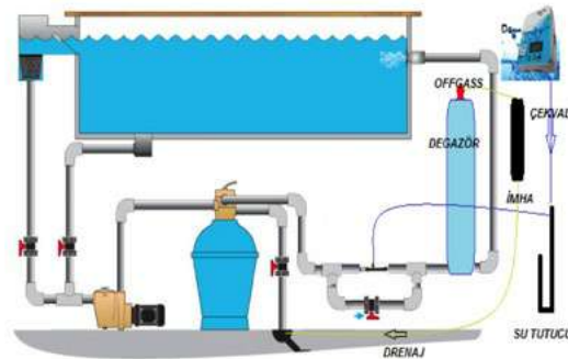
Dozon Midi Degazör Montaj Şeması Dozon Midi Degasors Installation Diagram
