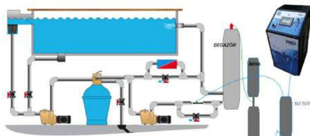
Dozon Maxi Degazör Montaj Şeması Dozon Maxi Degastor Assembly Diagram
