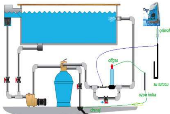
Dozon Mini Degazör Montaj Şeması Dozon Mini Degastor Assembly Diagram
